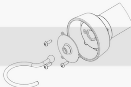
Vue éclatée crochet
